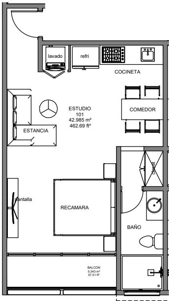
PLANTA ARQUITECTONICA
