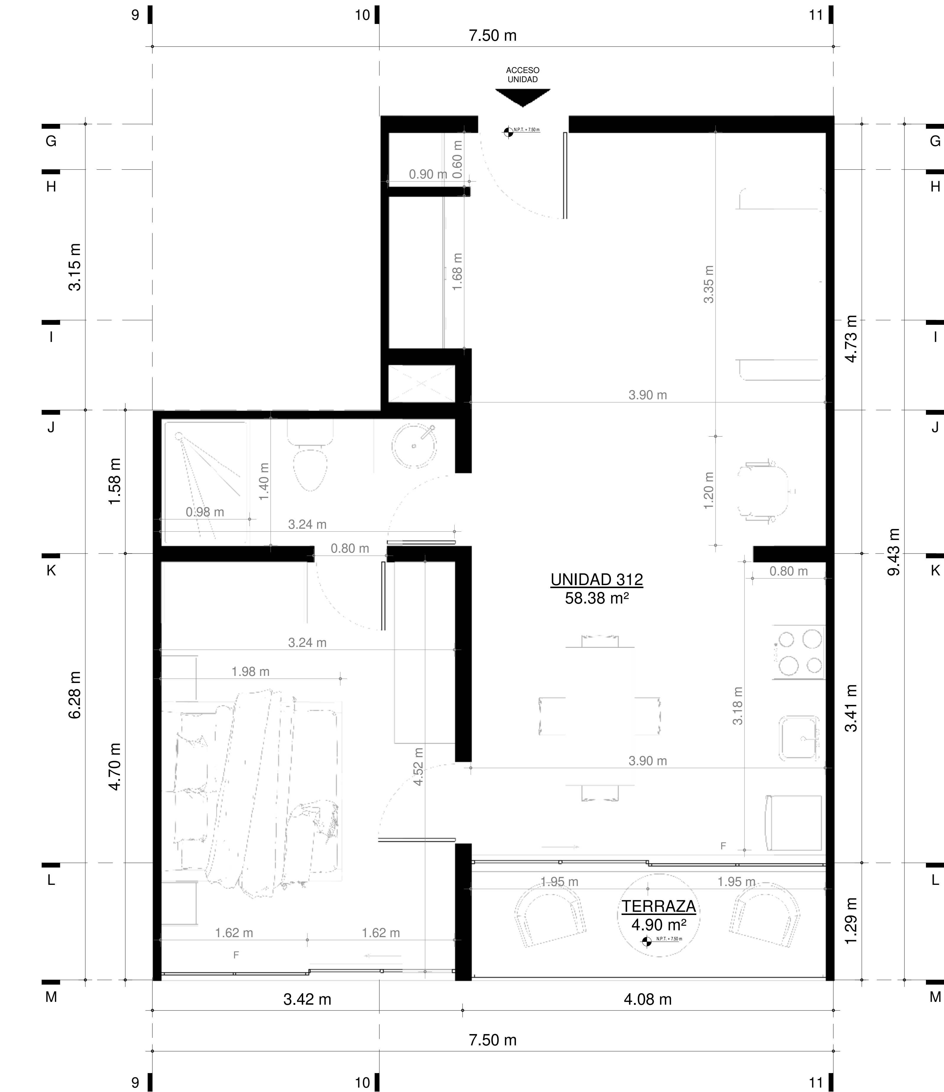
1 Unidad 312 1 : 25
