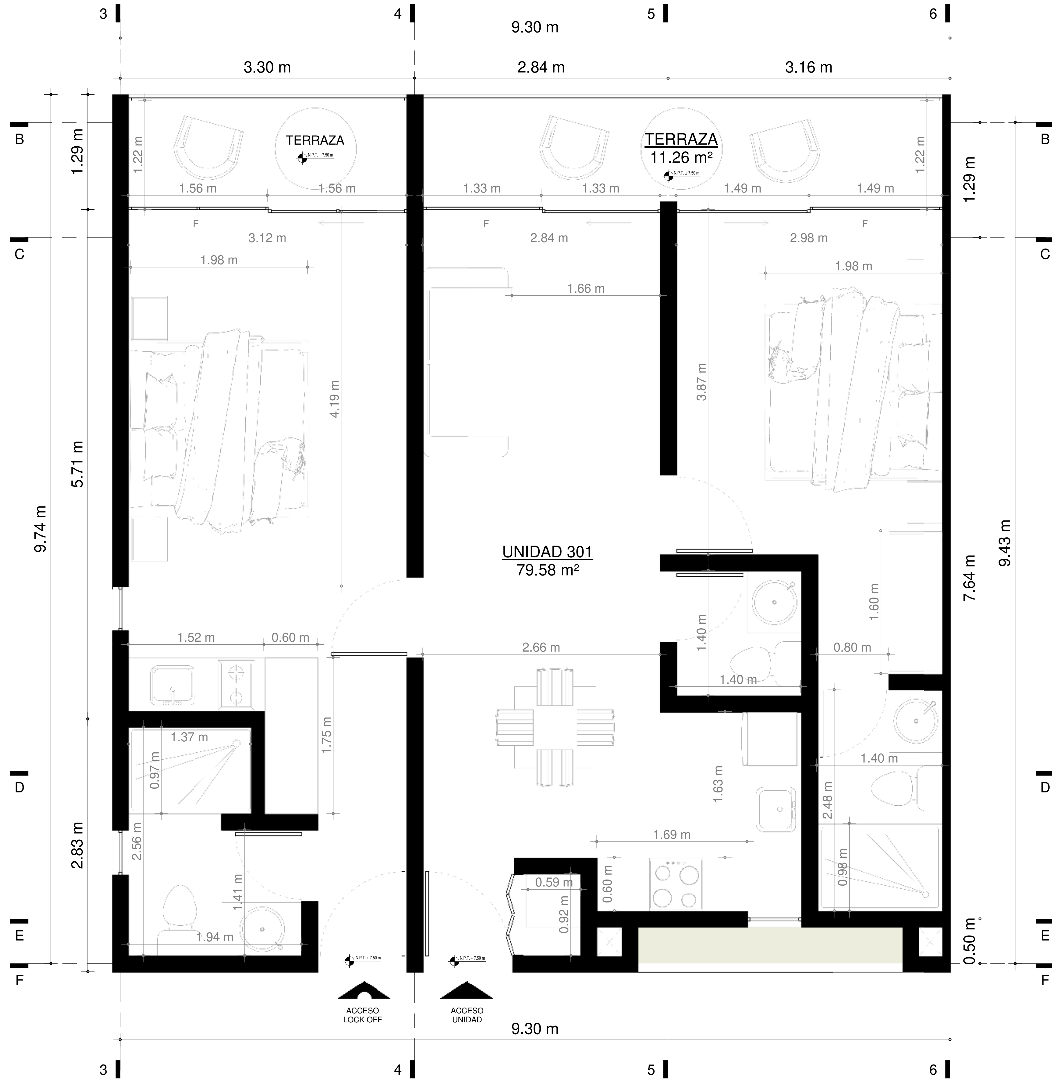
1 Unidad 301 1 : 25
