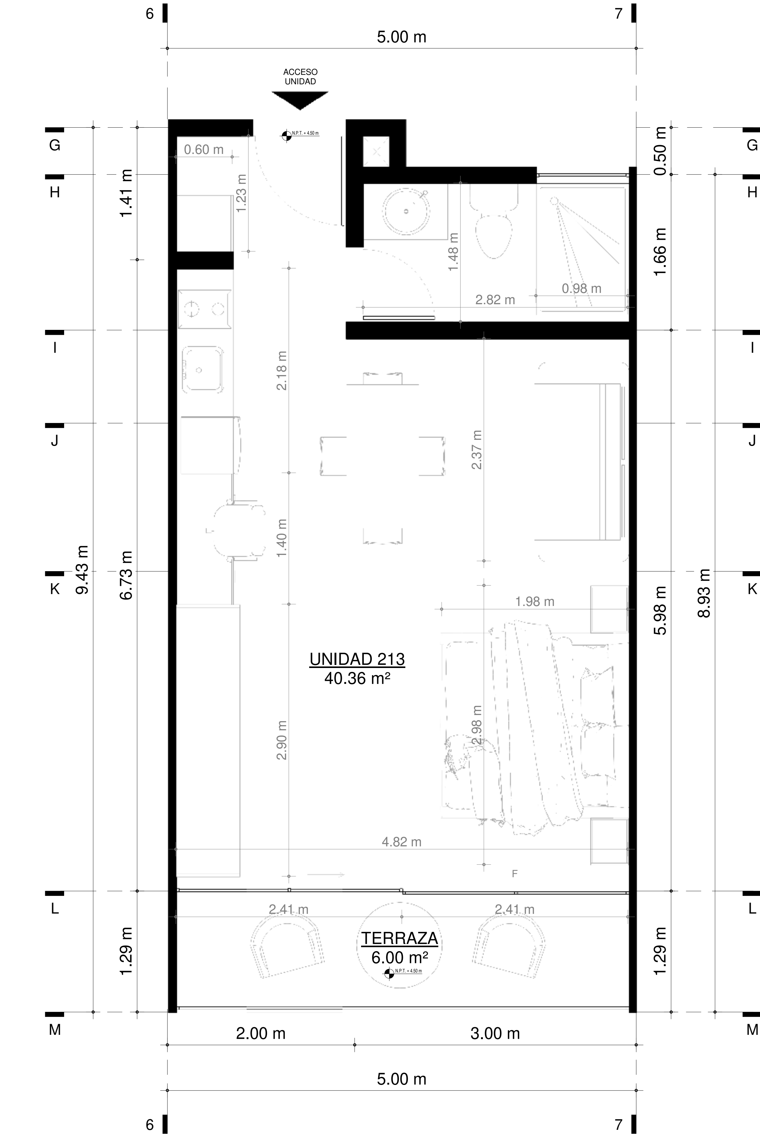
1 Unidad 213 1 : 25
