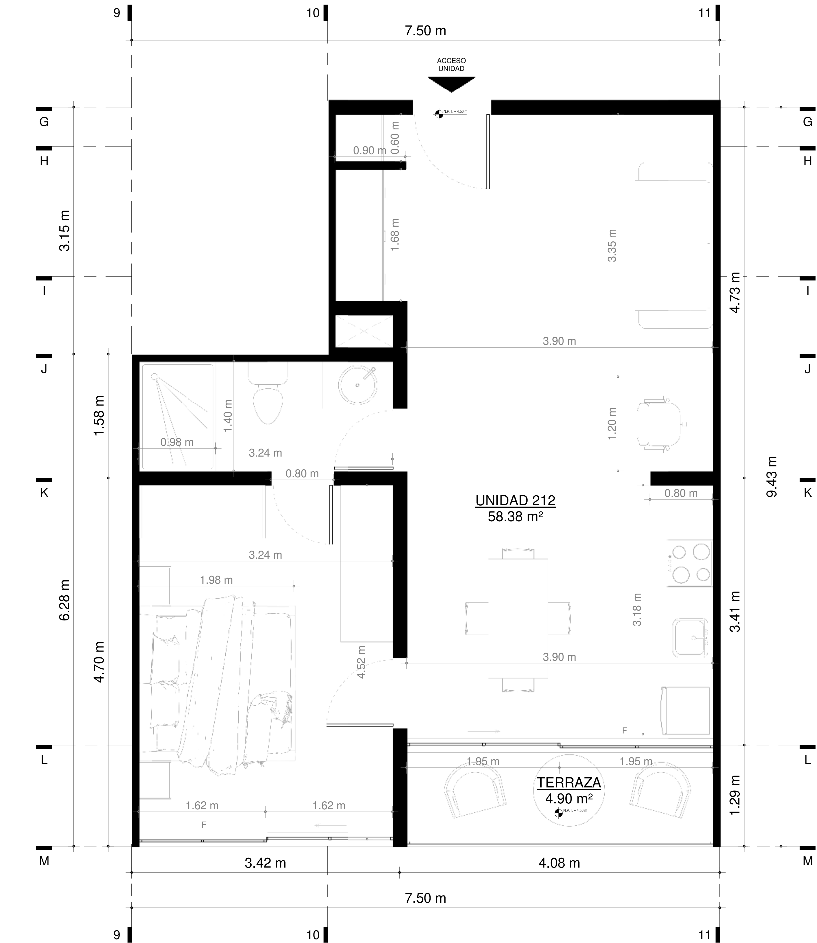
1 Unidad 212 1 : 25
