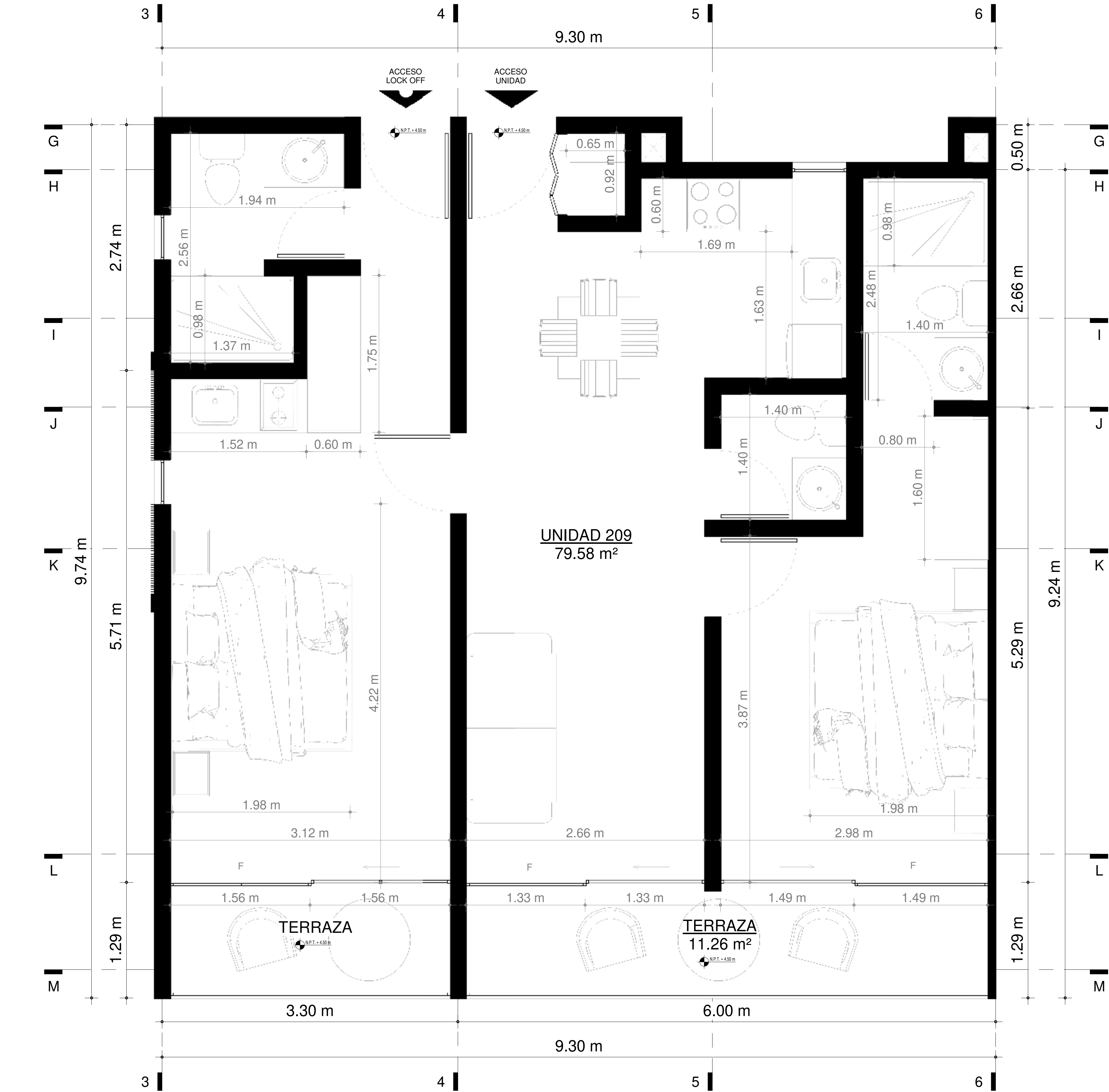
1 Unidad 209 1 : 25
