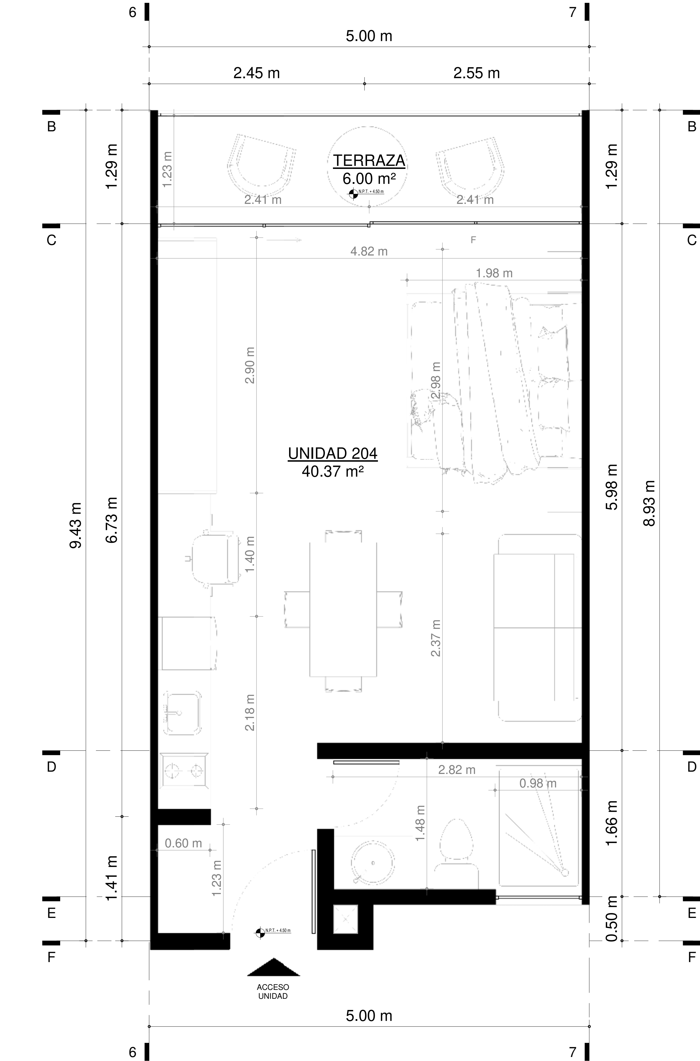
1 Unidad 204 1 : 25
