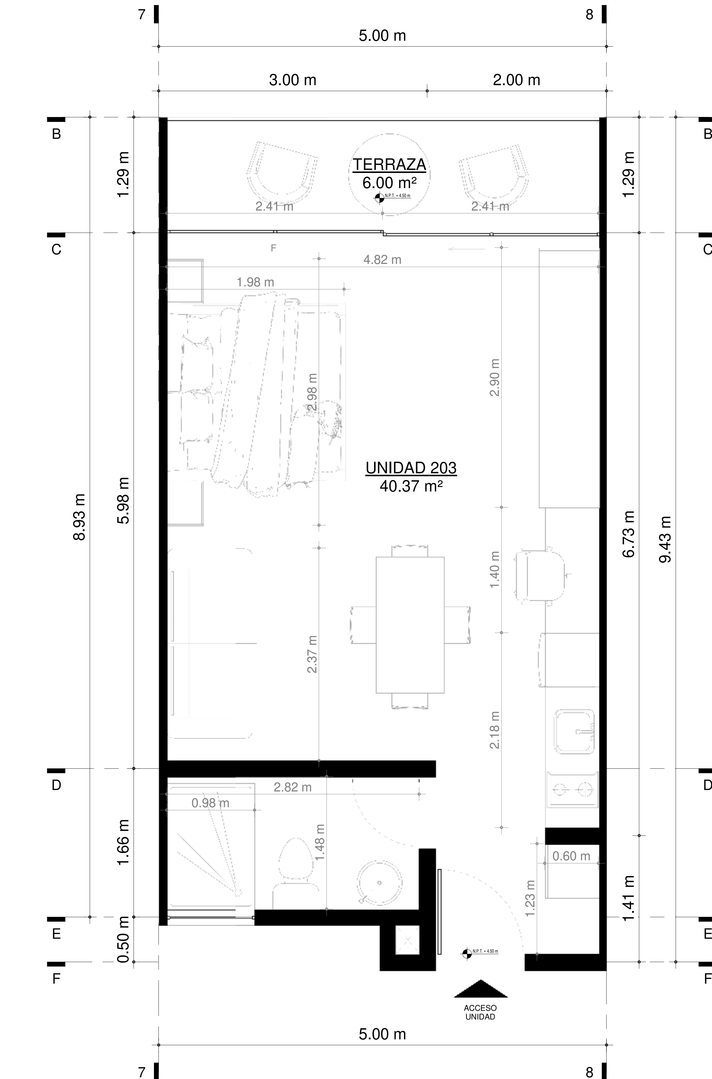
1 Unidad 203 1 : 25
