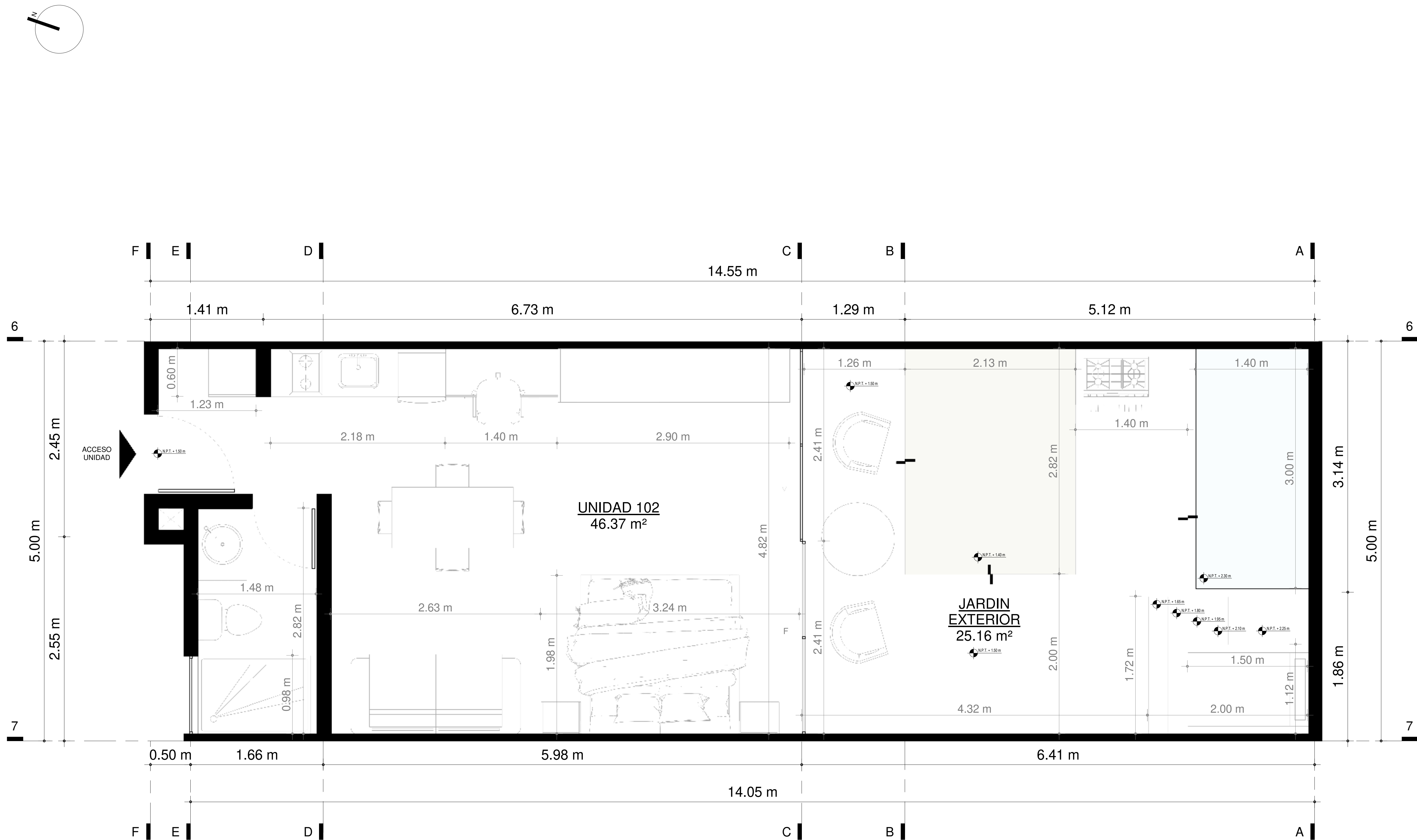
Unidad 102 1 : 25
