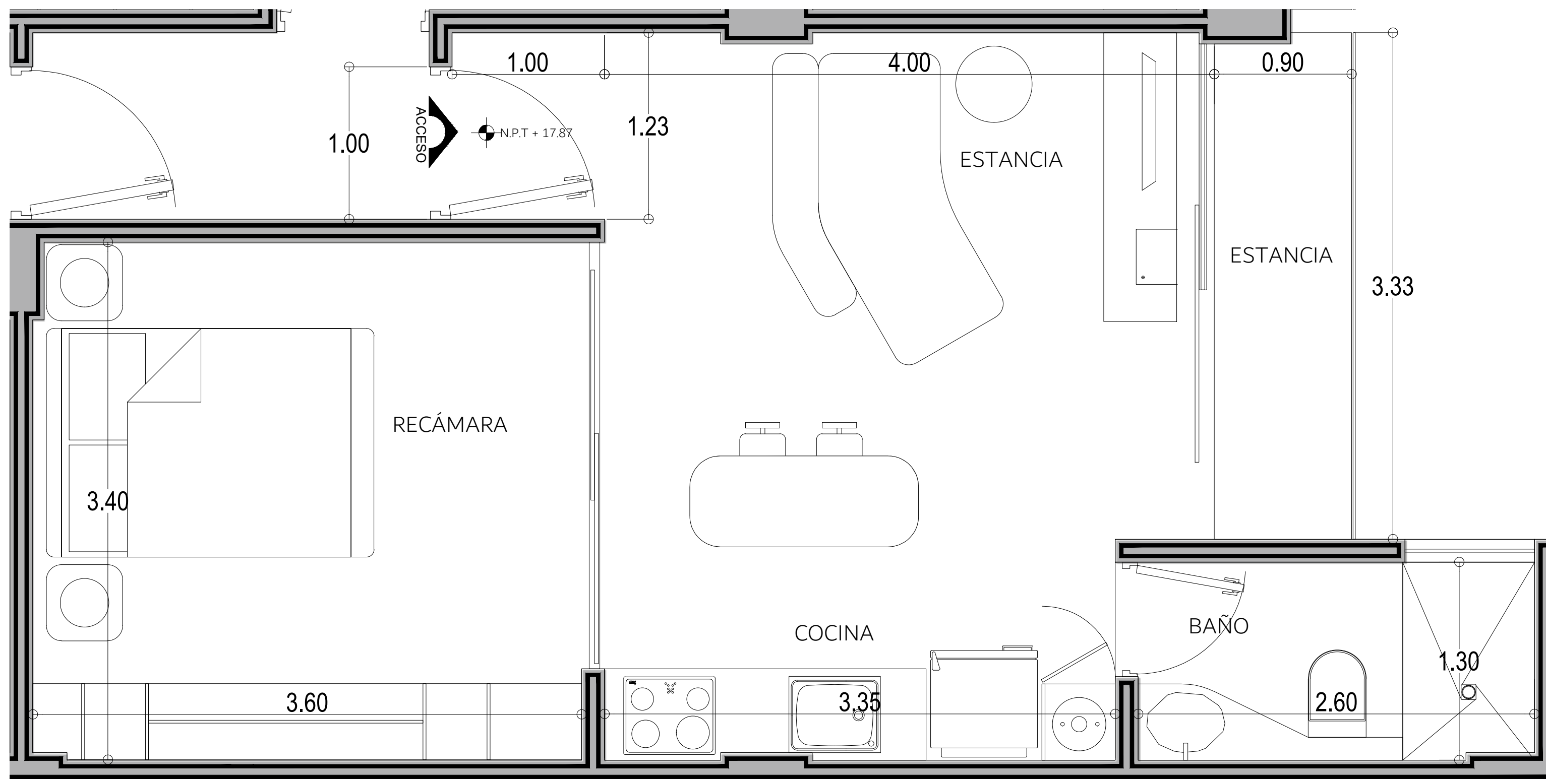
PLANTA ARQUITECTÓNICA DEPARTAMENTO C503 ESCALA 1:10
