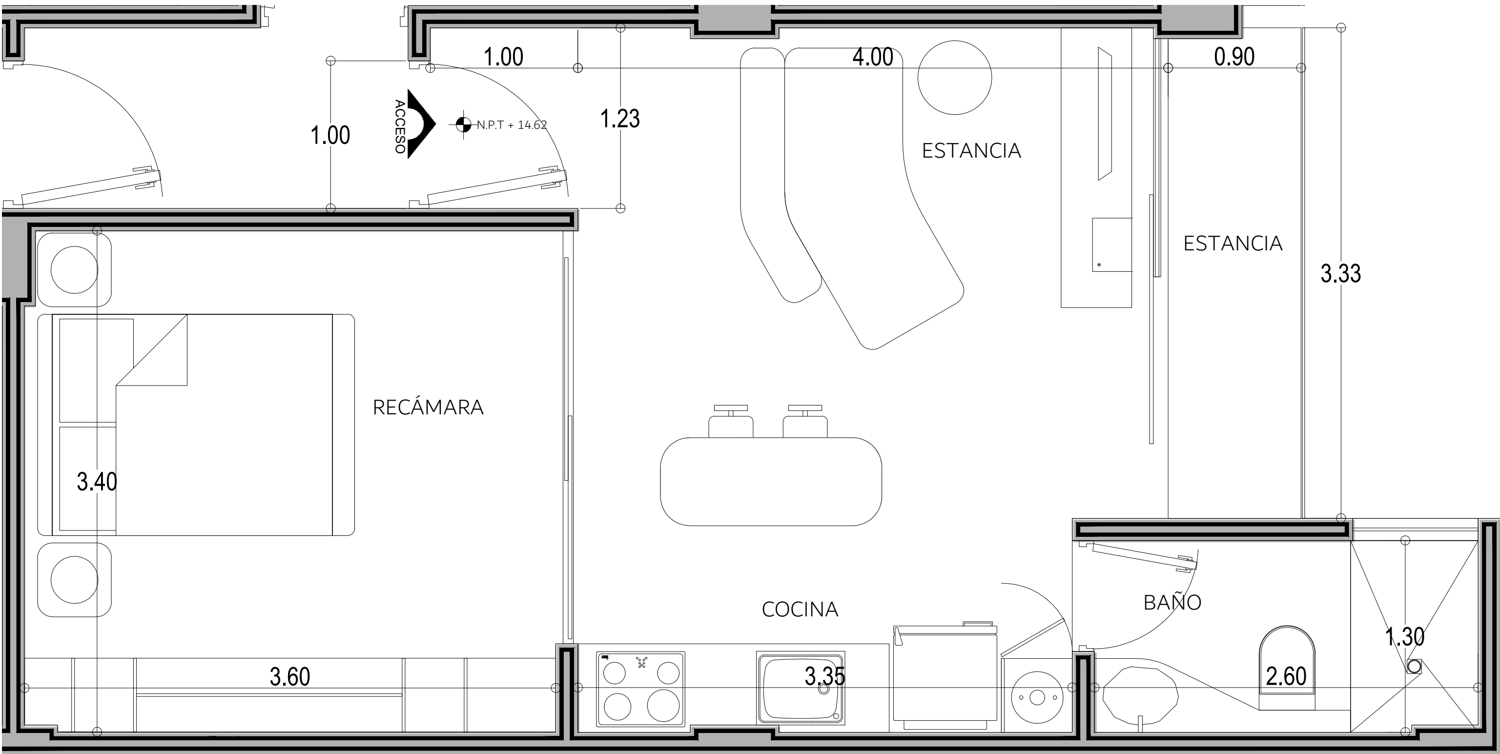
PLANTA ARQUITECTÓNICA DEPARTAMENTO C403 ESCALA 1:10
