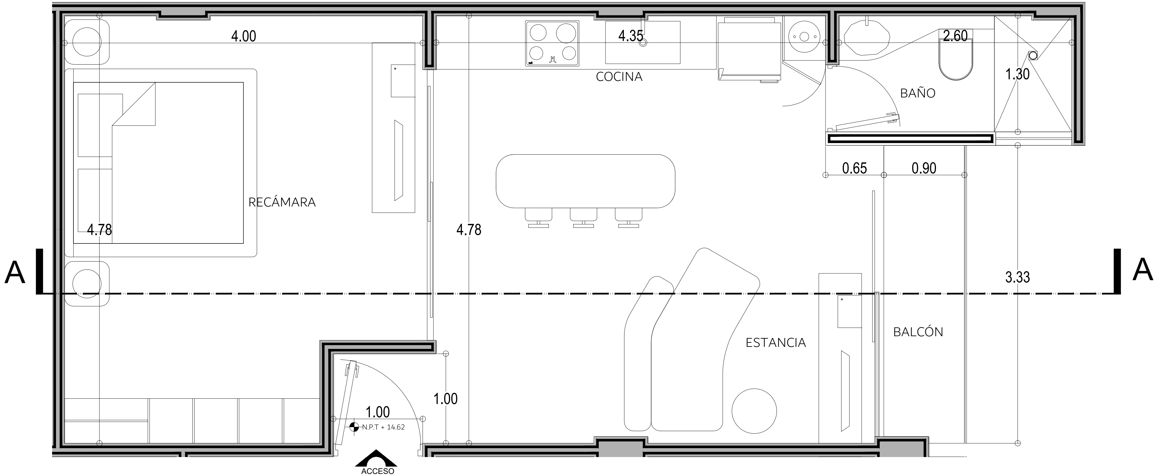
PLANTA ARQUITECTÓNICA DEPARTAMENTO B402 ESCALA 1:10
