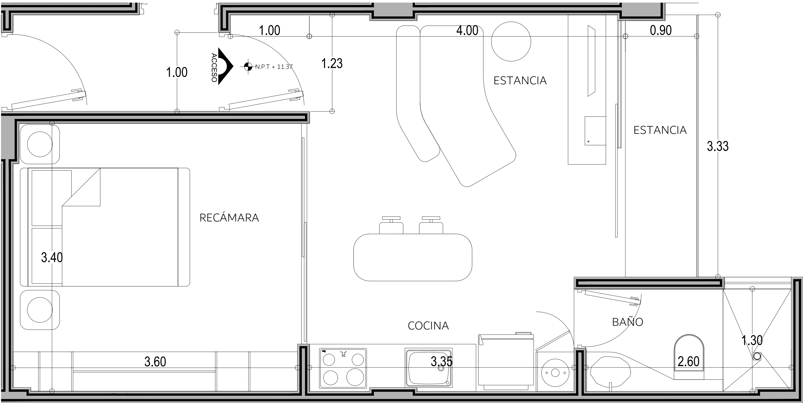
PLANTA ARQUITECTÓNICA DEPARTAMENTO C303 ESCALA 1:10
