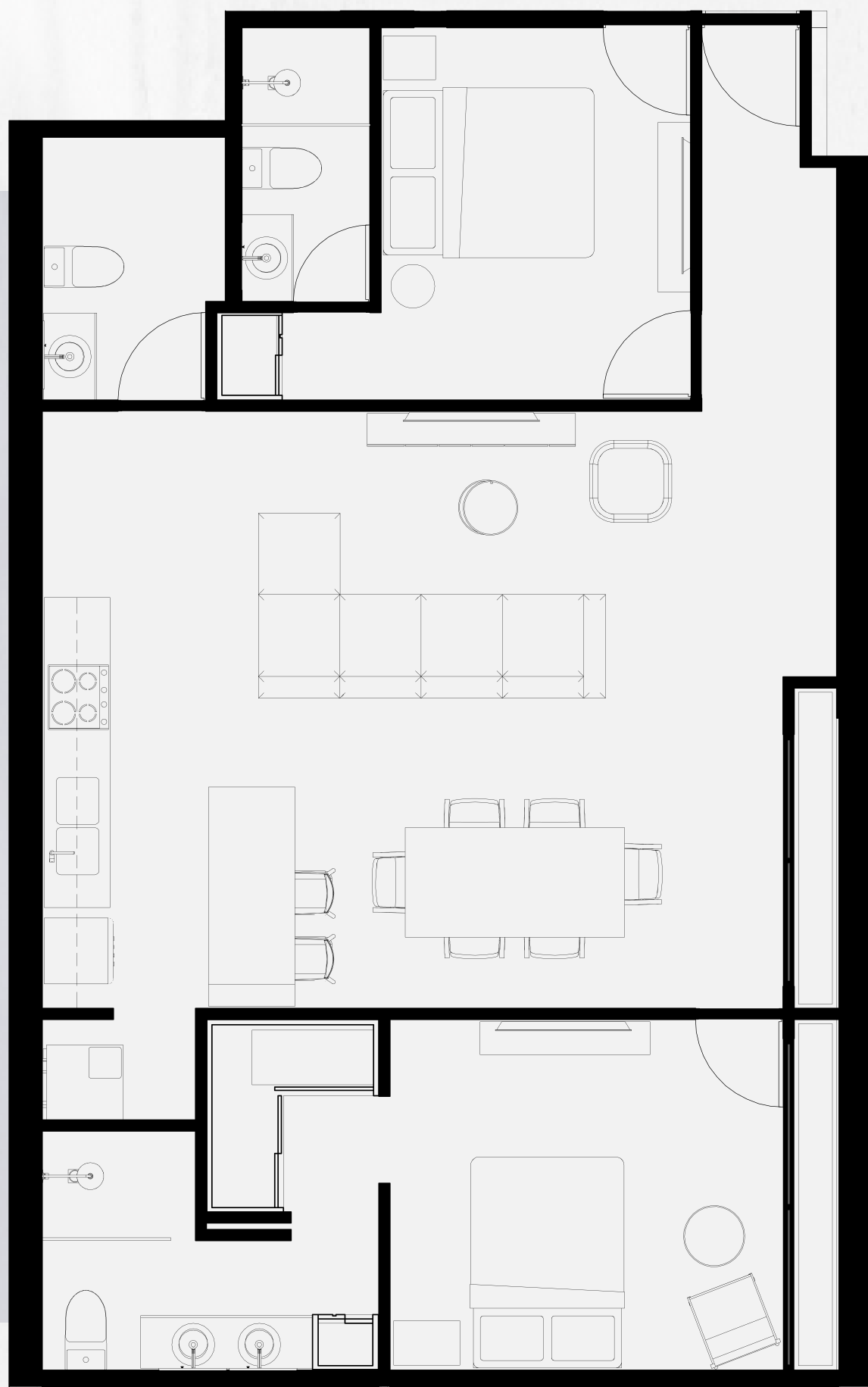
Planta arquitectónica 2D
