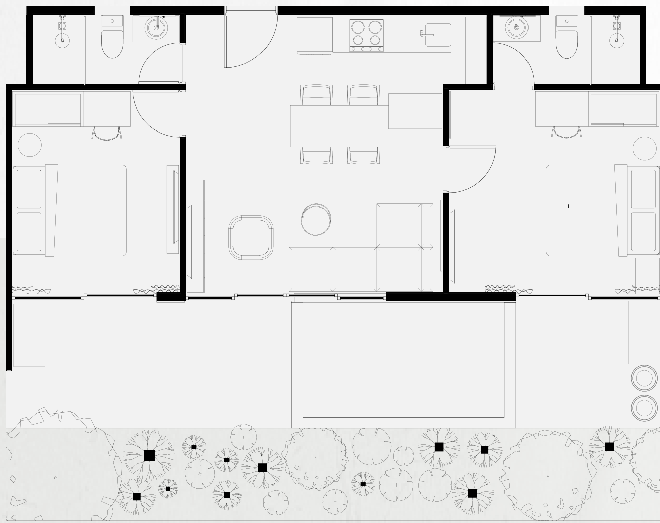
Planta arquitectónica 2D
