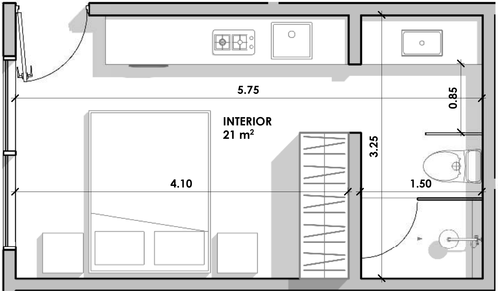
DEPARTAMENTO 106-A 21 m 2
