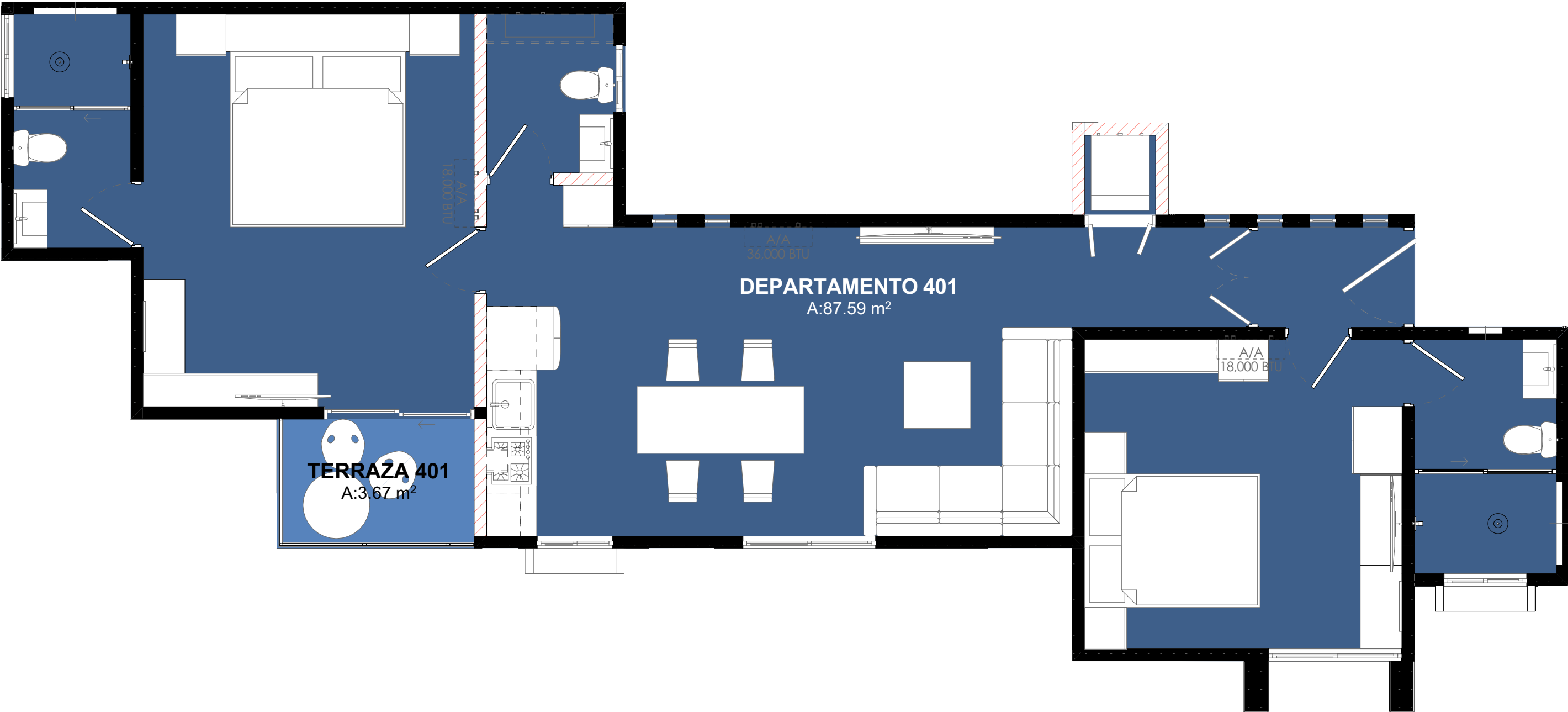
3. NIVEL 1 - DEPARTAMENTO 401 1:50
