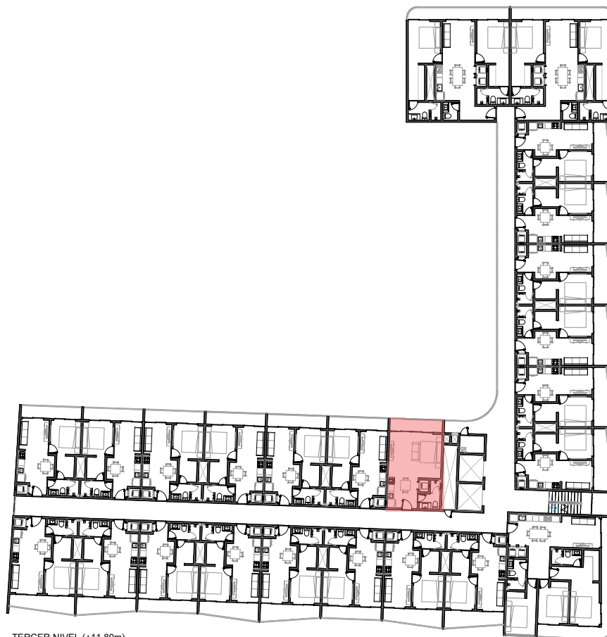
TERCER NIVEL (+11.80m)
