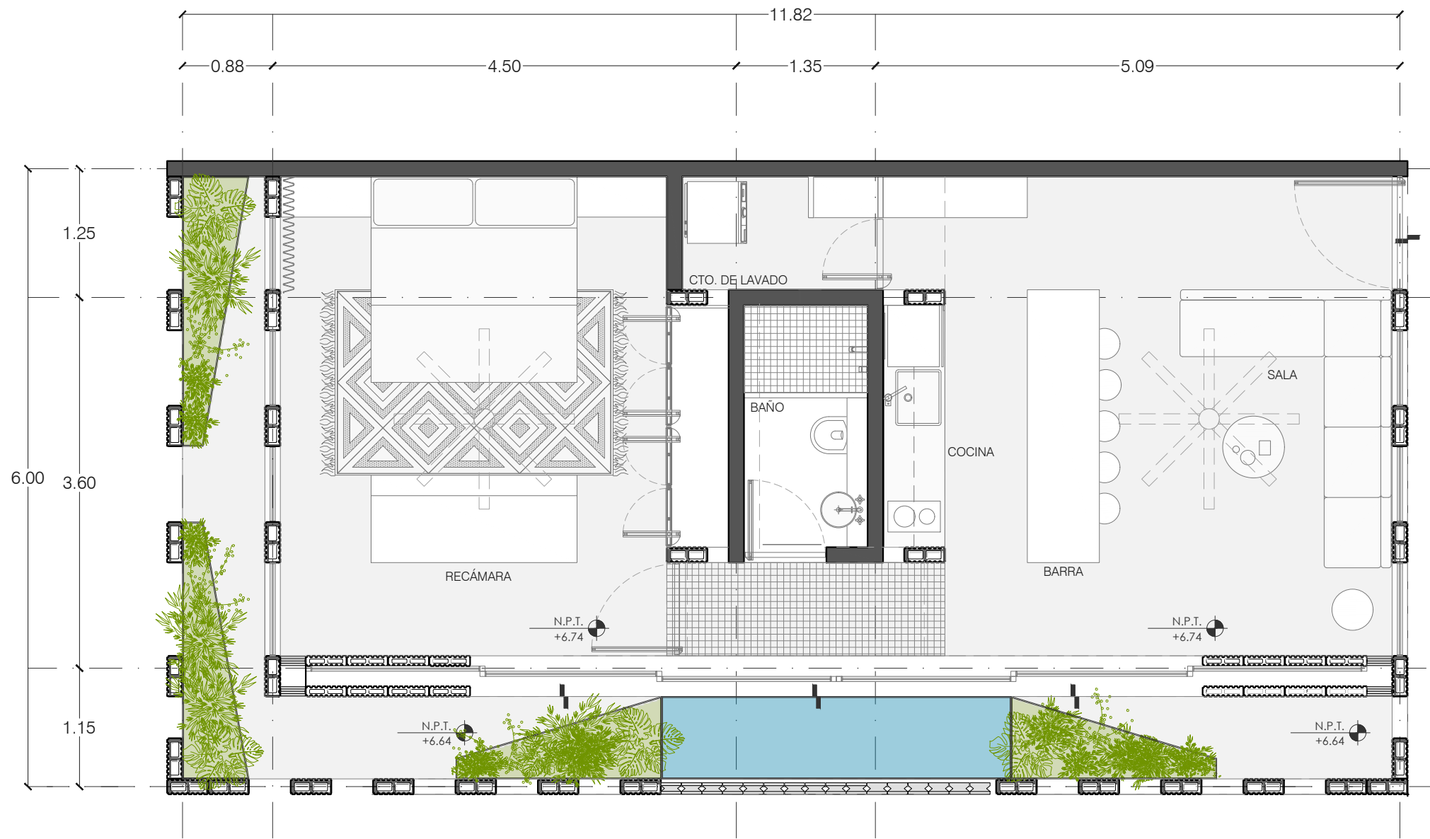
1. Planta Arquitectonica Green Suite 15 1:50
