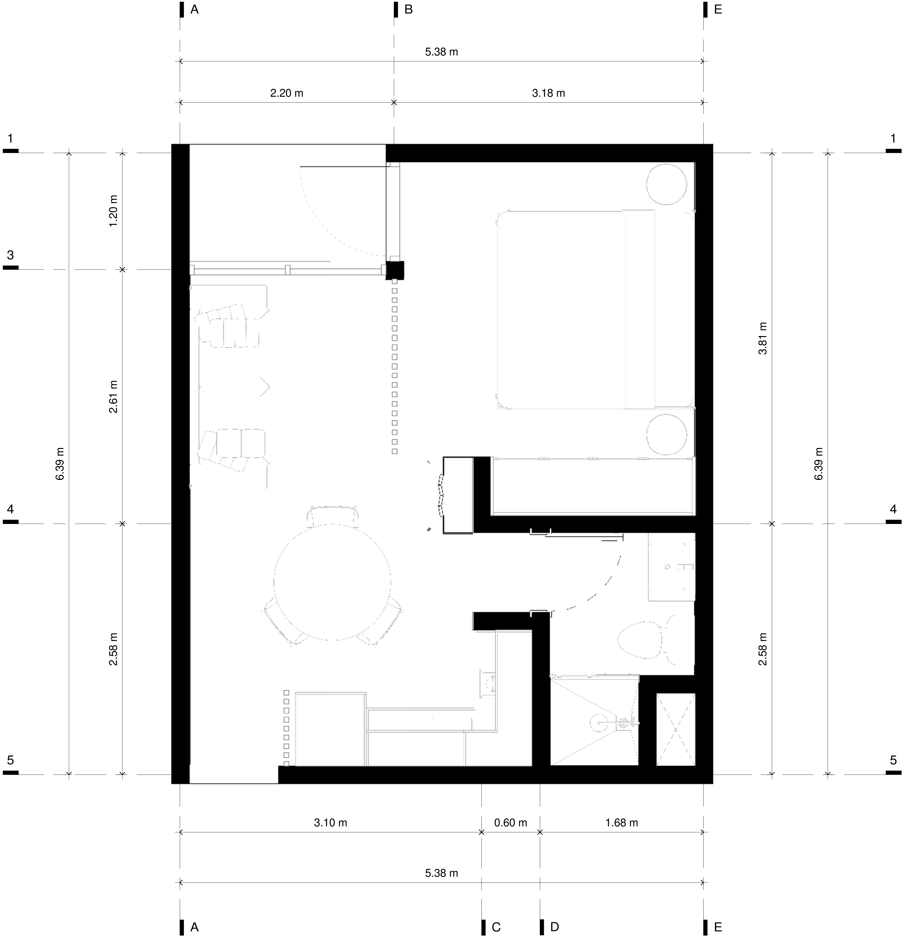
1 STUDIO TIPO 03 1 : 20
