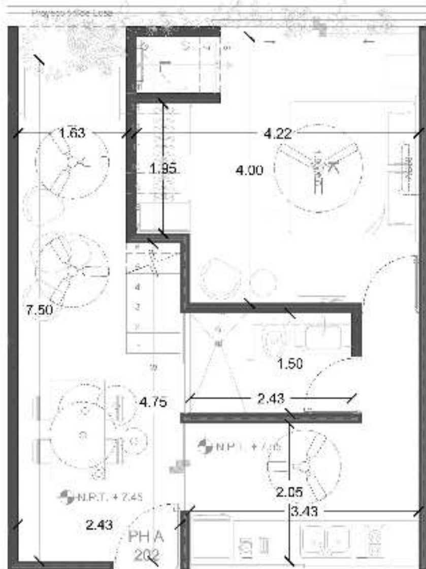
PENTHOUSE 202 TIPO A – Planta Baja
