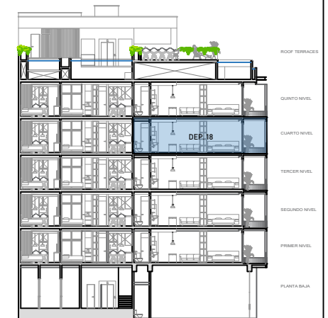
CORTE SECCION I SOBRE CALLE 78
