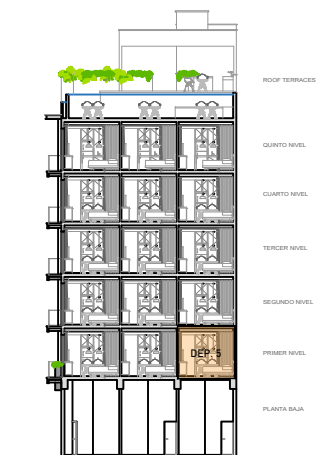
CORTE SECCION 2 SOBRE 5a AVENIDA
