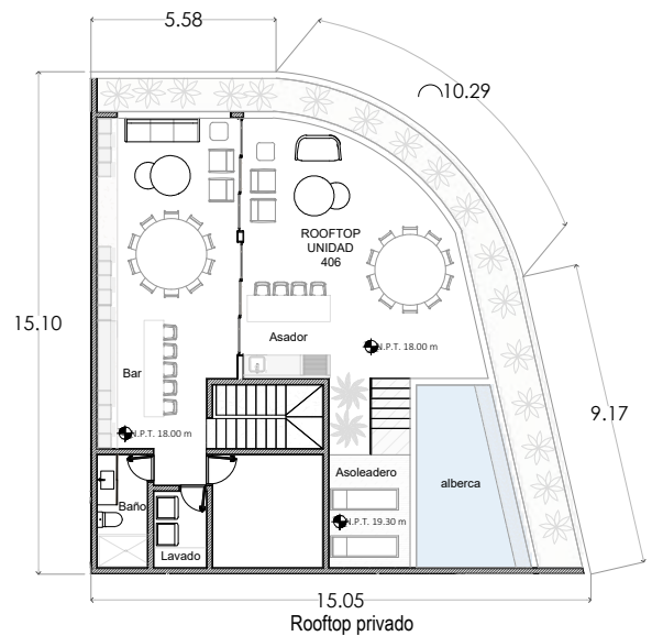
Planta Rooftop
