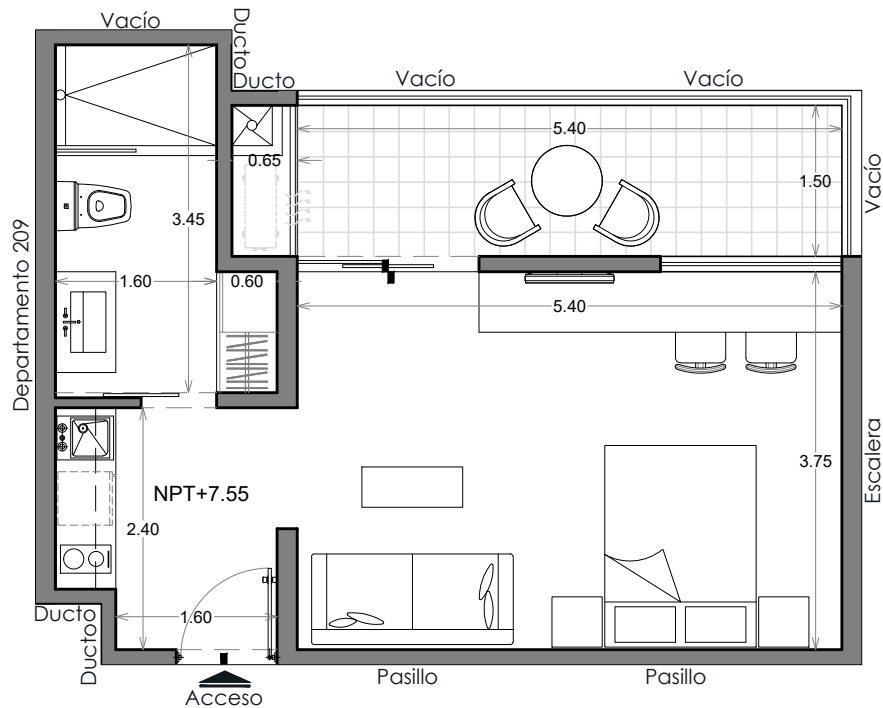
Planta Arquitectónica Esc. 1:75
