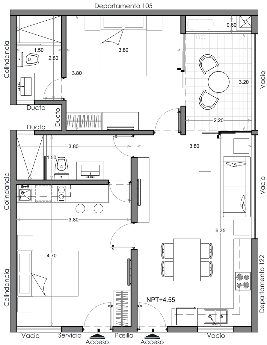
Planta Arquitectónica Esc. 1:75
