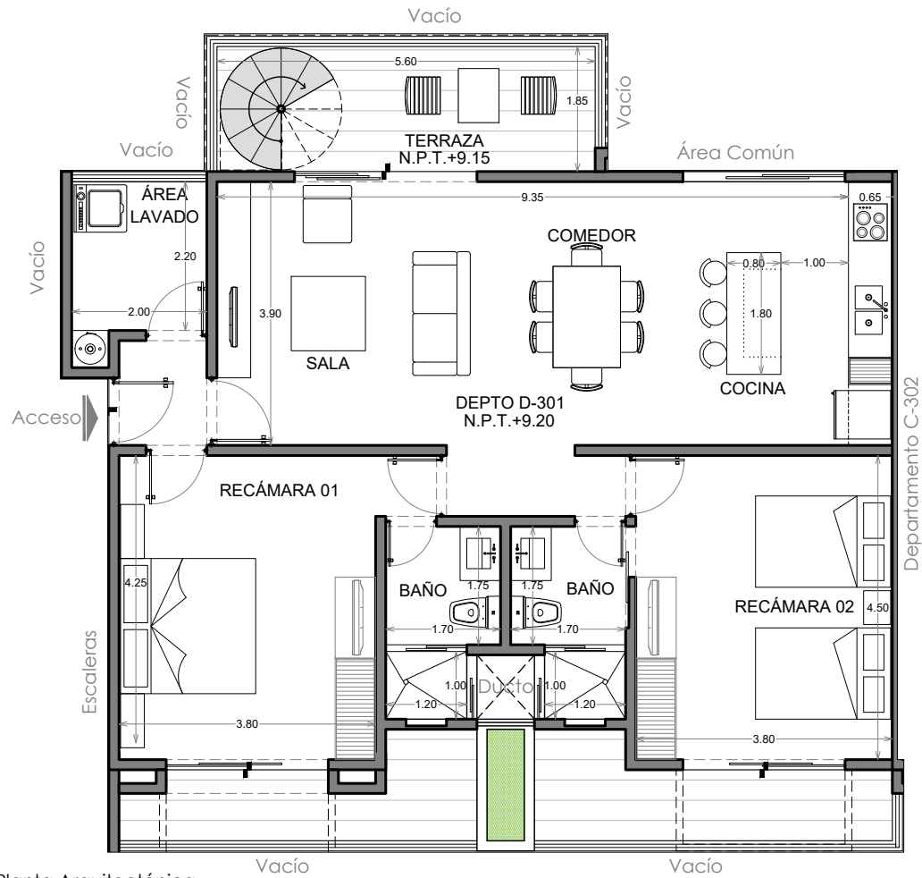
Planta Arquitectónica Esc. 1:100
