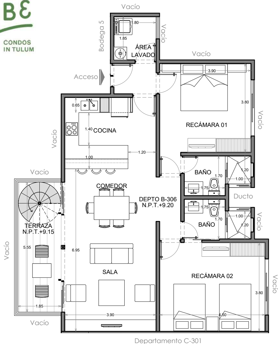
Planta Arquitectónica Esc. 1:100
