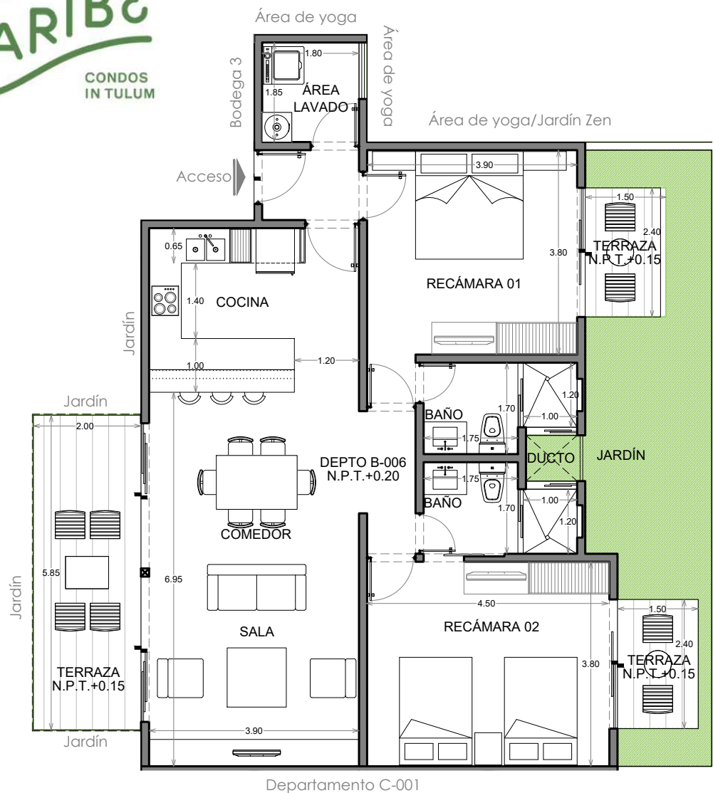
Planta Arquitectónica Esc. 1:100
