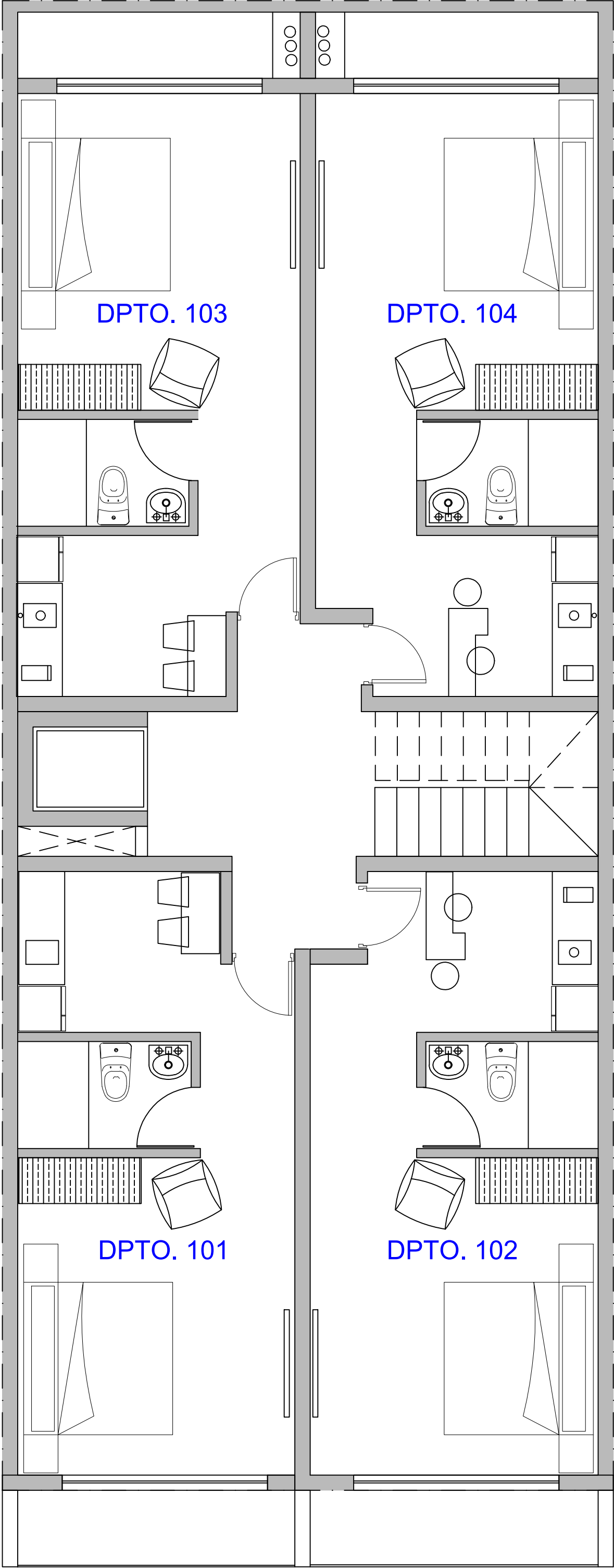
PLANTA 1ER NIVEL
