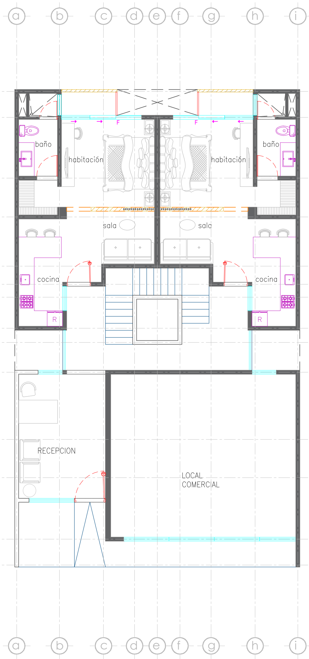
PLANTA BAJA
