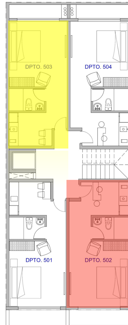
PLANTA 5TO NIVEL
