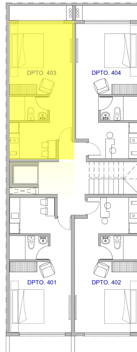
PLANTA 4TO NIVEL
