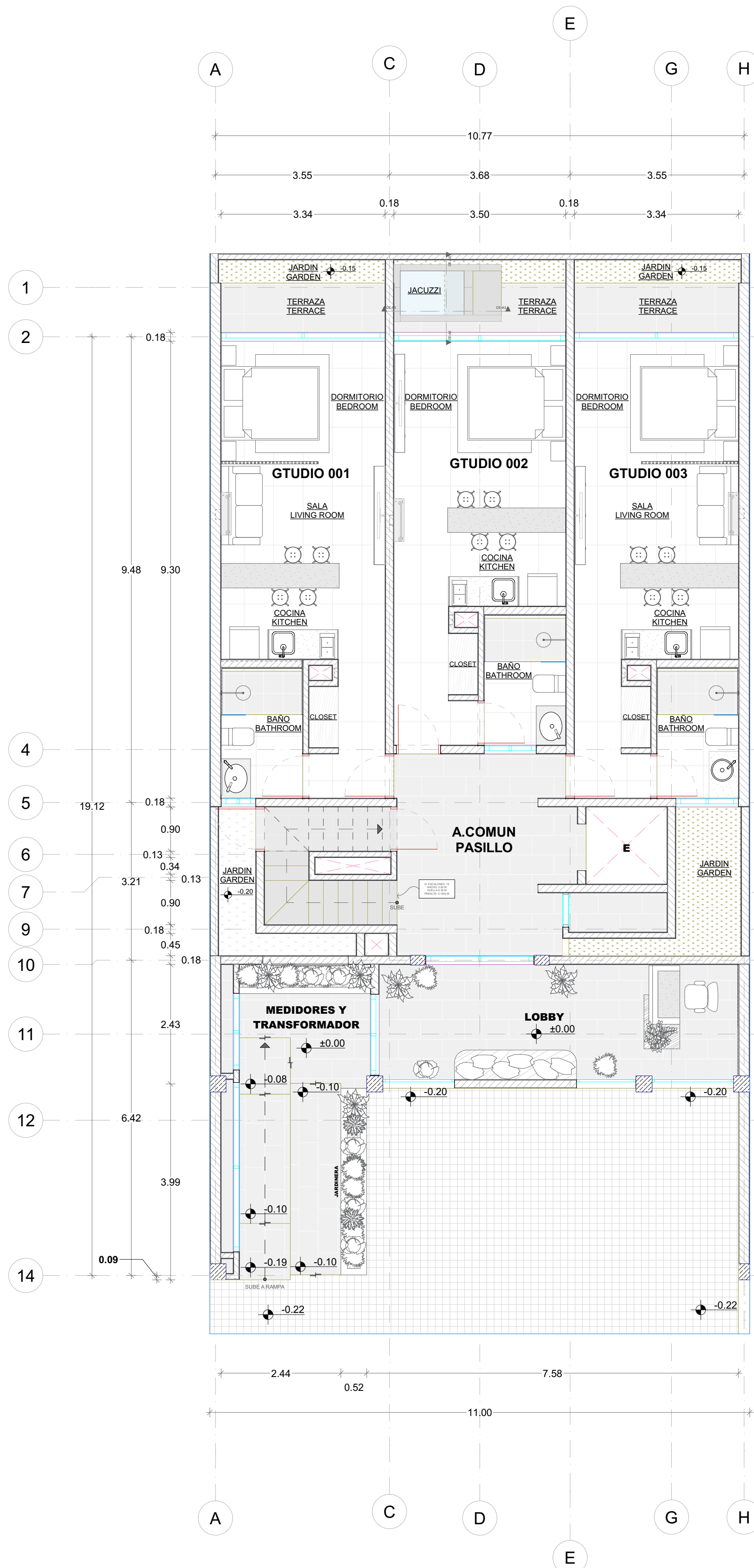
1 PLANTA BAJA ARQUITECTONICO S/N
