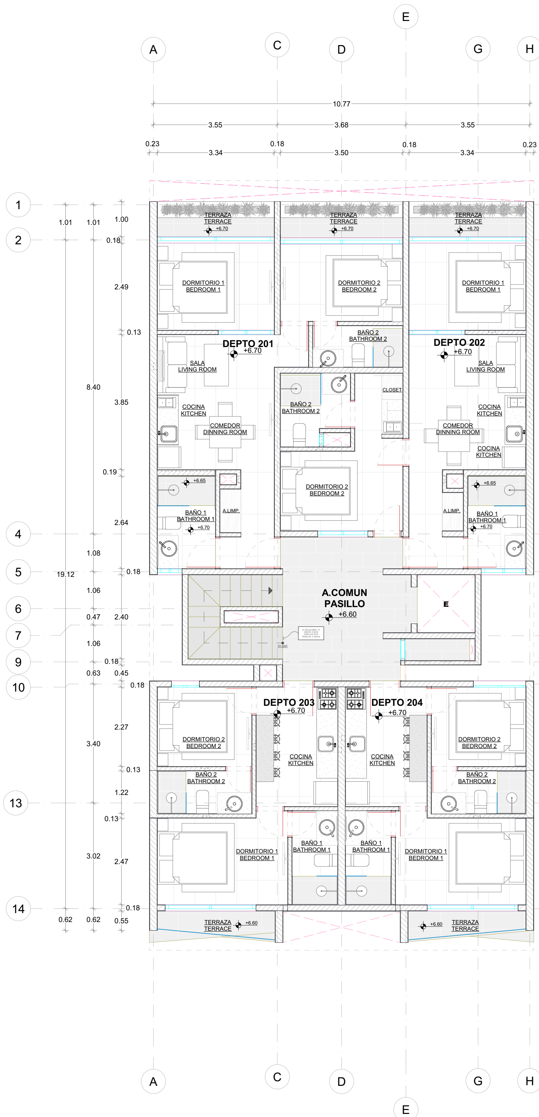
1 SEGUNDO NIVEL ARQUITECTONICO S/N
