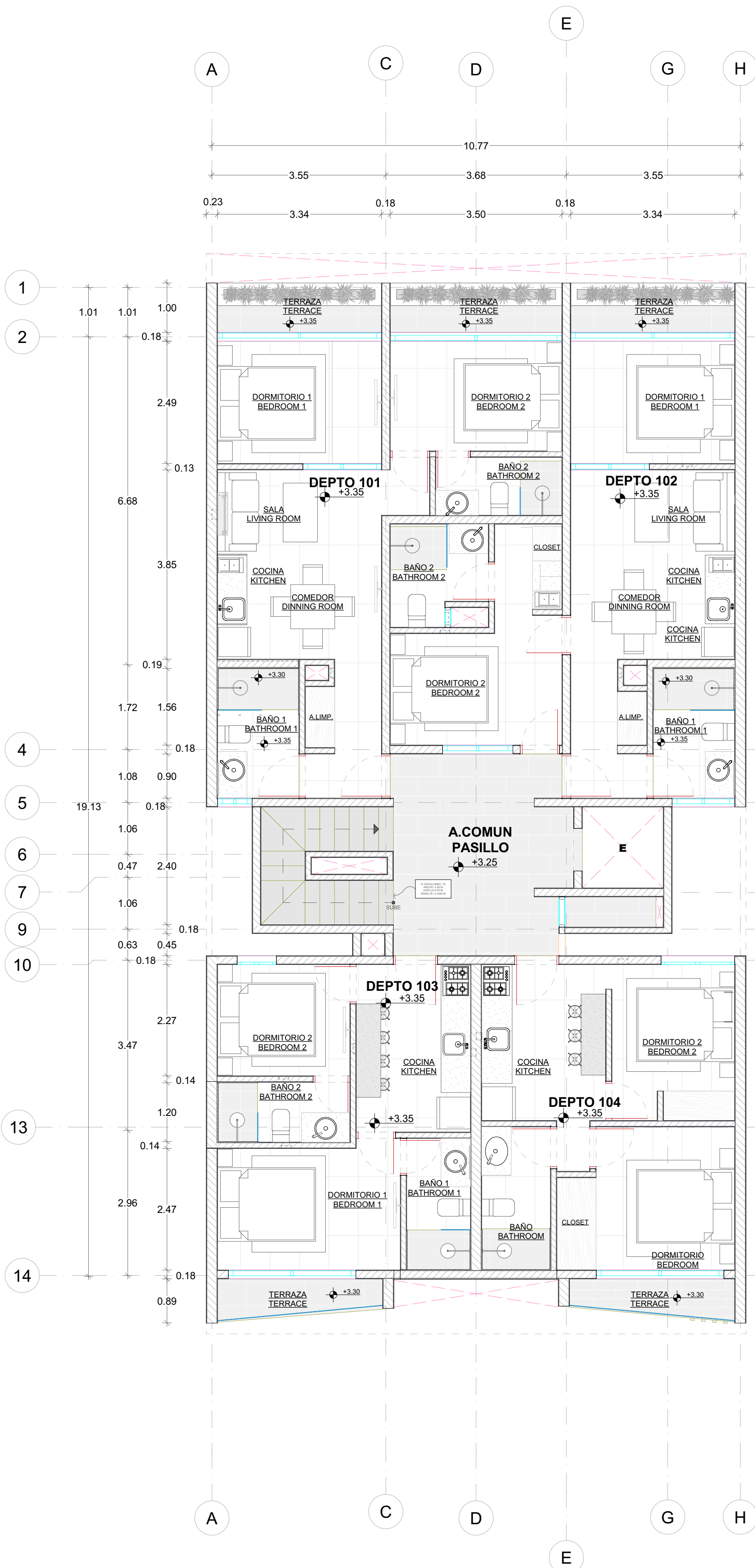
2 PRIMER NIVEL ARQUITECTONICO S/N
