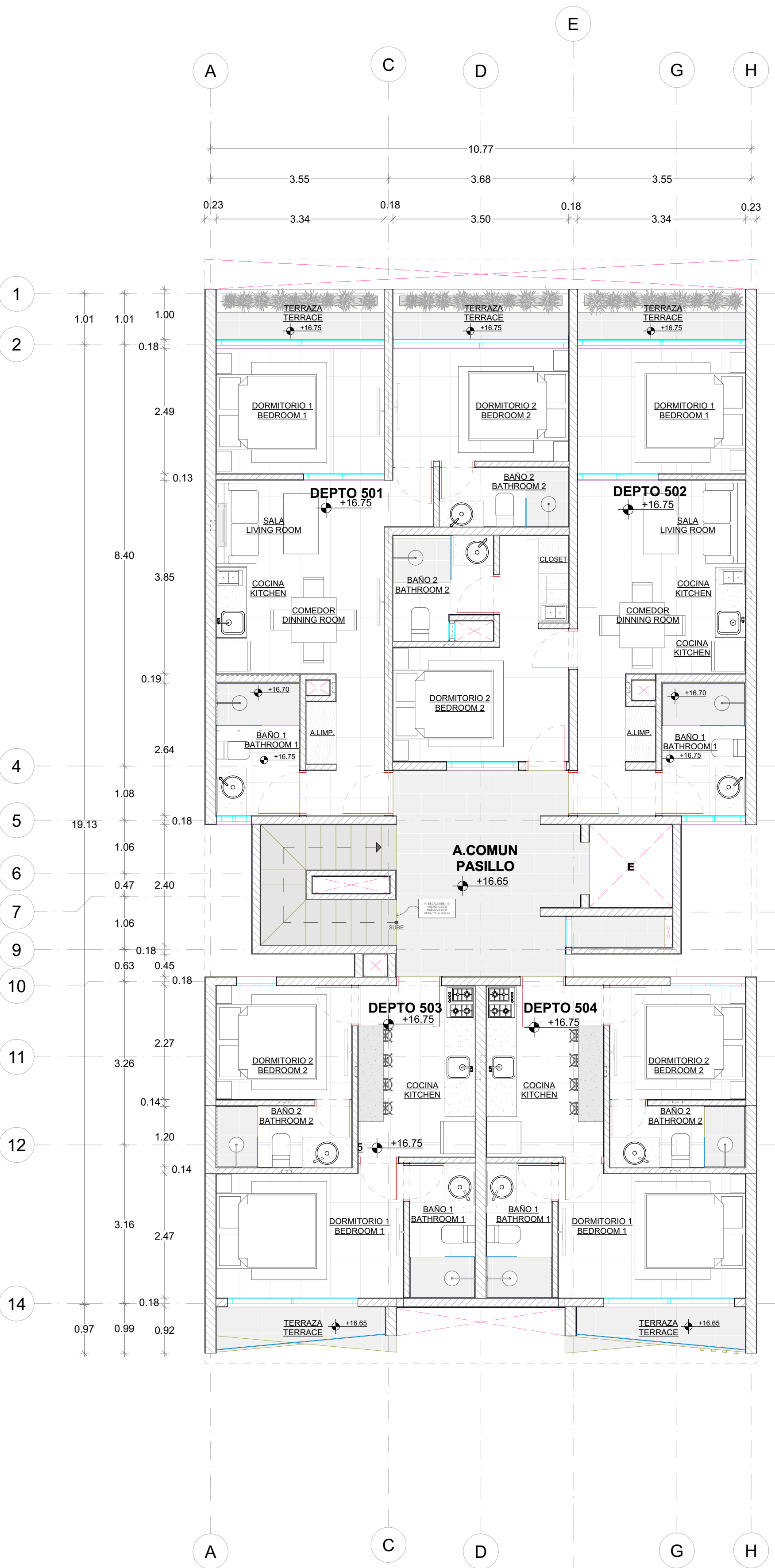
2 QUINTO NIVEL ARQUITECTONICO S/N
