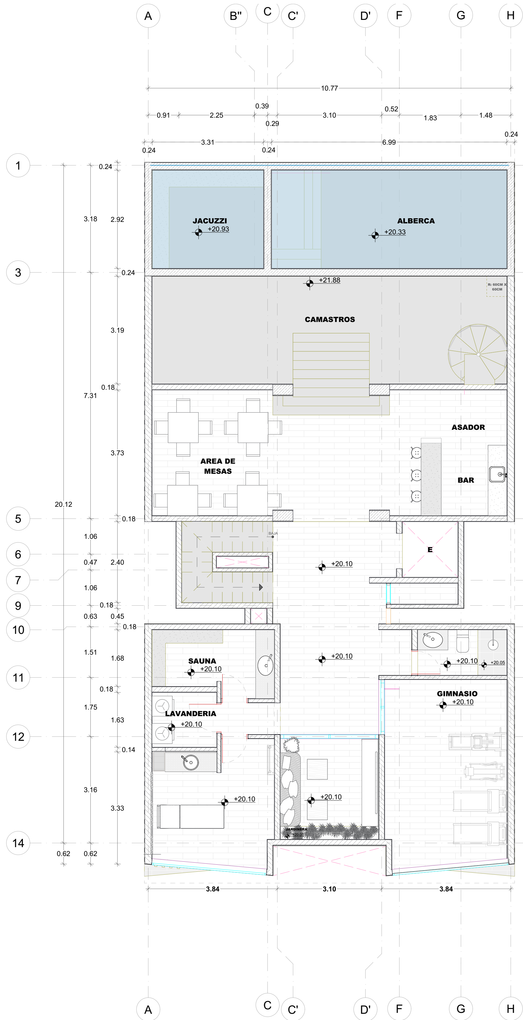
1 ROOF TOP ARQUITECTONICO S/N
