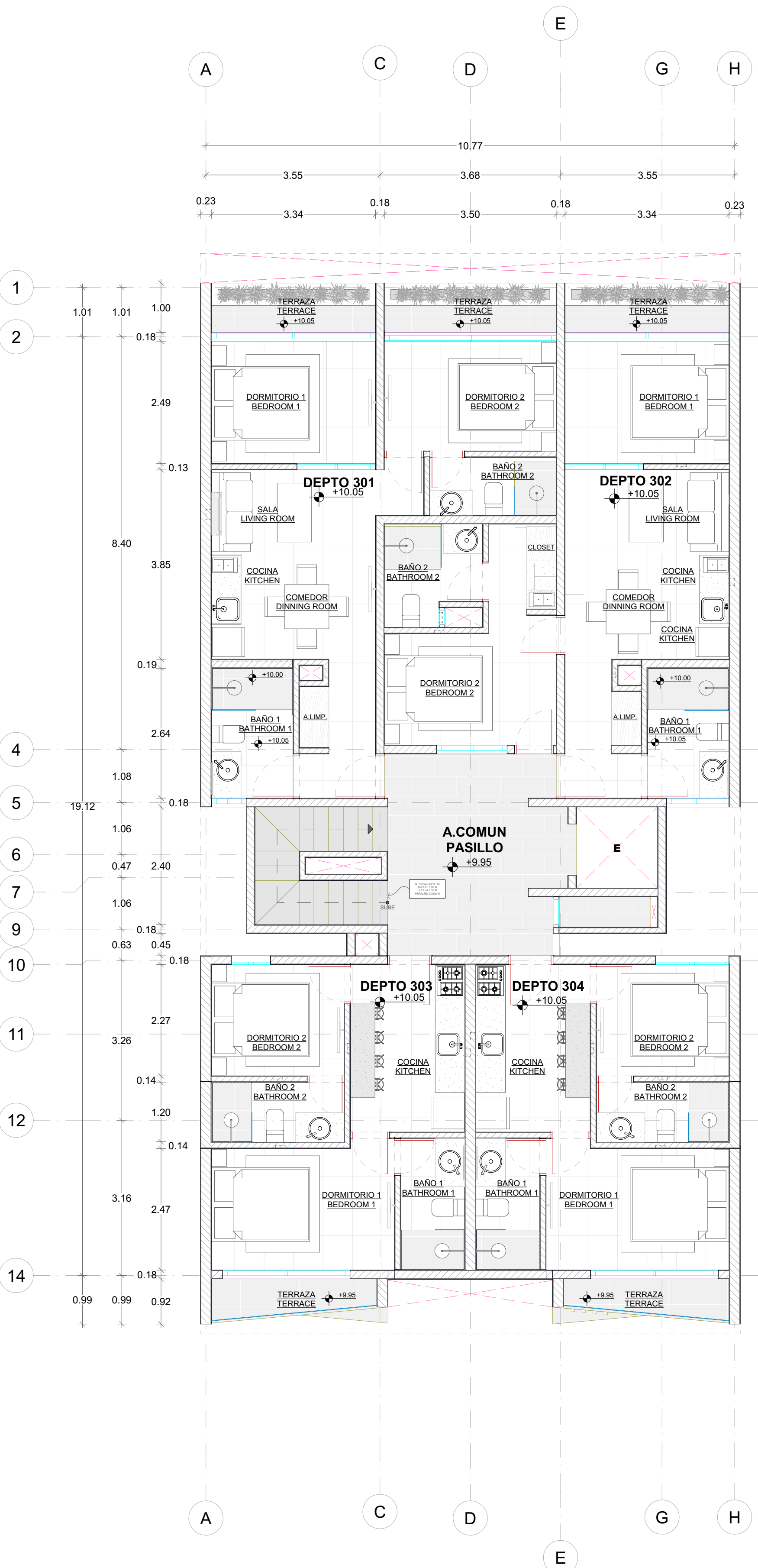
2 TERCER NIVEL ARQUITECTONICO S/N
